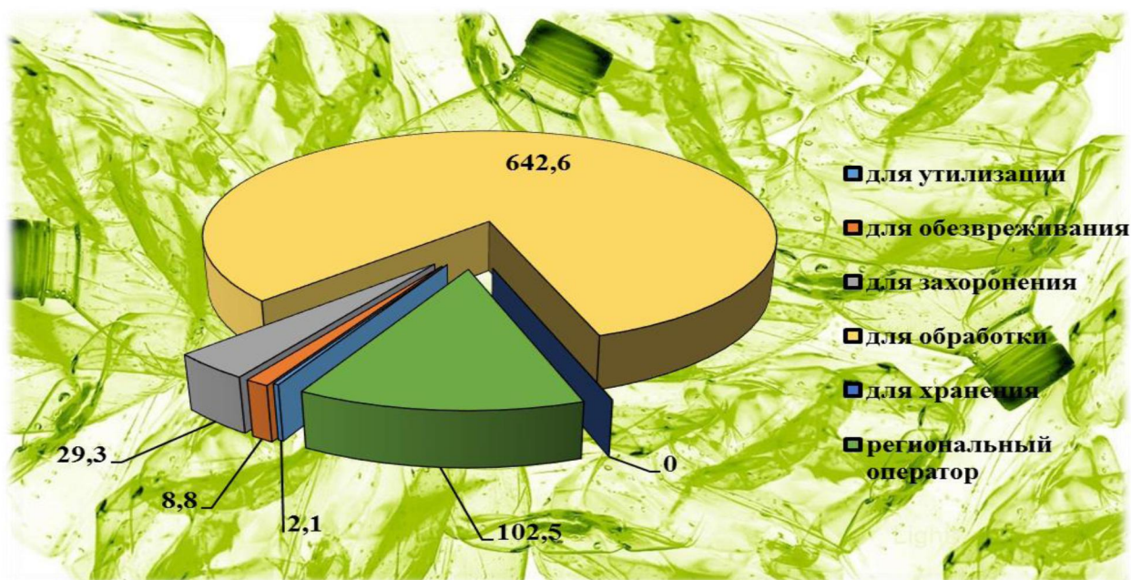
Диаграмма 4. Передача отходов другим организациям, тонн/год
