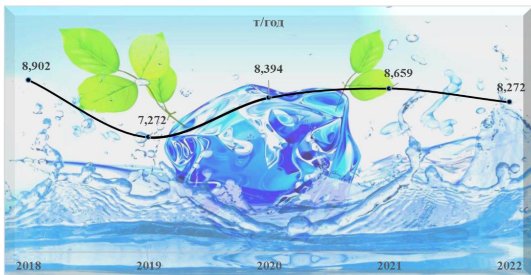
Диаграмма 2. Валовые сбросы загрязняющих веществ, поступающие с ливневыми стоками в р. Ельцовка – 2, тонн/год.
