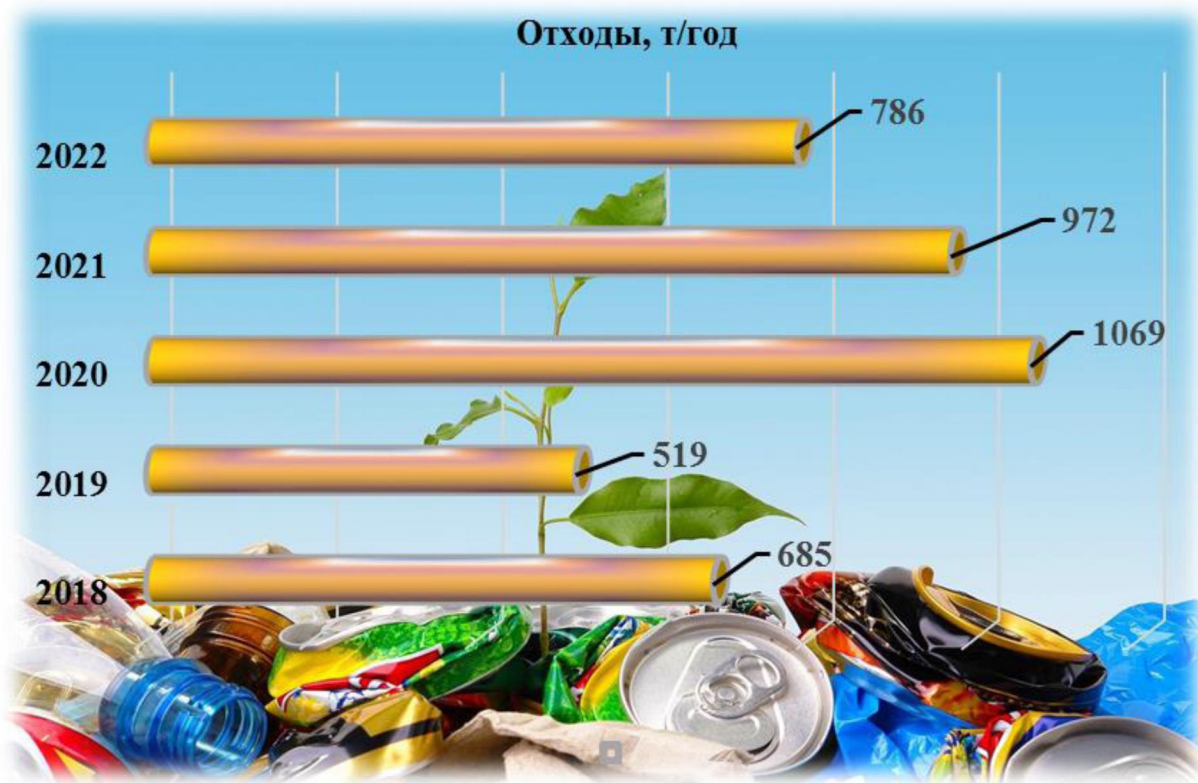
Диаграмма 5. Образование отходов производства и потребления
