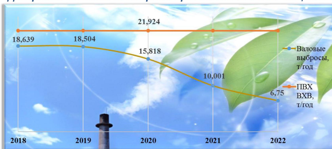
Диаграмма 3. Валовые выбросы вредных химических веществ
