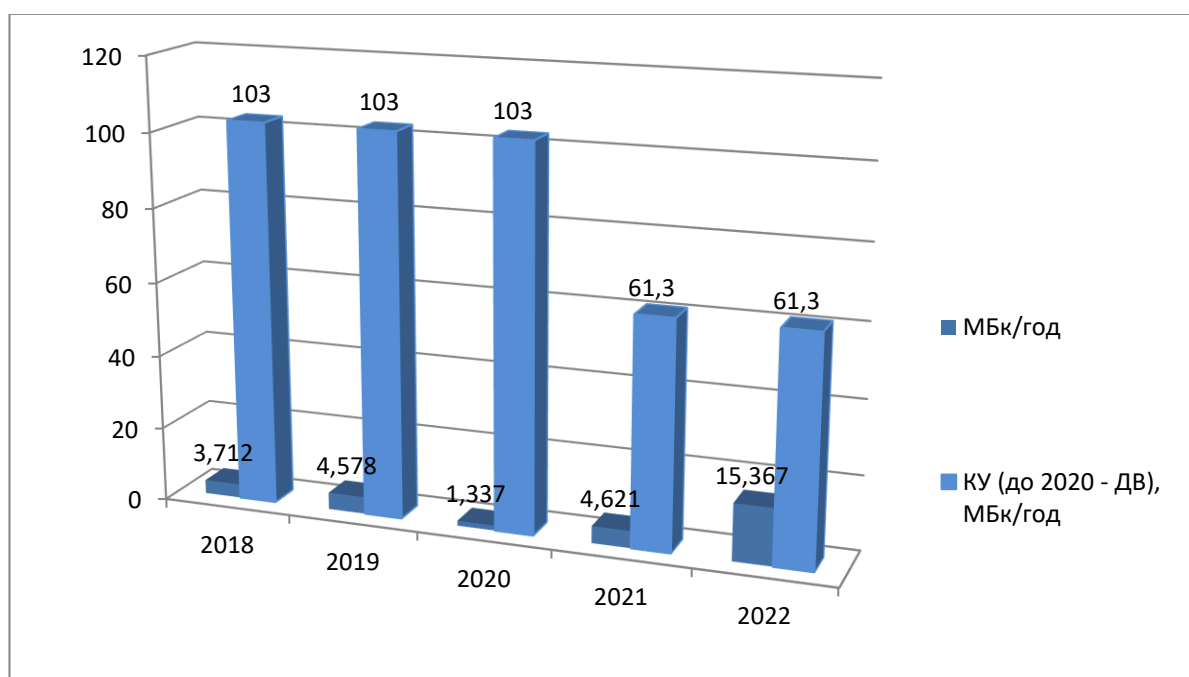
Диаграмма 5. Динамика выброса радионуклидов в атмосферу в НПК – Сергиево-Посадского филиала ФГУП «РАДОН»
