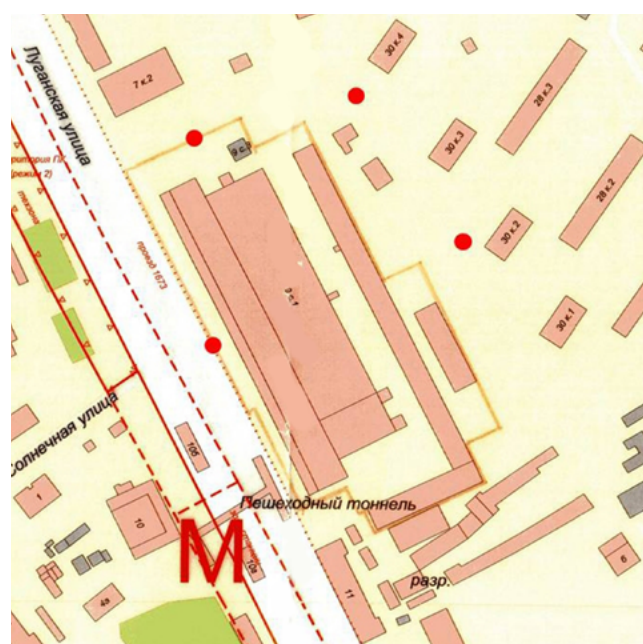
Карта-схема расположения точек контроля на границе СЗЗ пл. «Царицыно»
