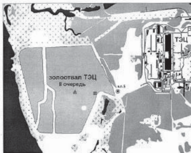
Б.1 - Схема расположения мест отбора проб приземного атмосферного воздуха, подземных вод и почвы в районе расположения золоотвала II-й очереди
