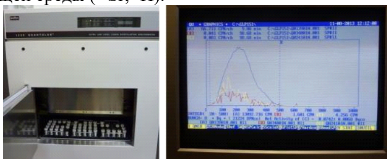
Рисунок 14 – Низкофоновый жидкостно-сцинтилляционный радиометр-спектрометр "Quantulus 1220" и набираемый спектр
