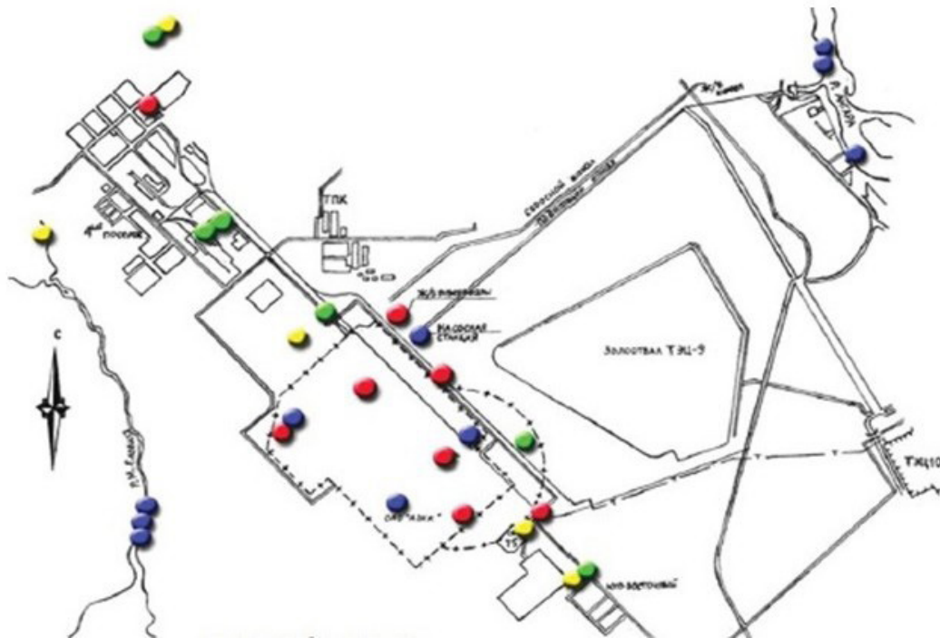
Рисунок 2. КАРТА-СХЕМА КОНТРОЛЯ ОБЪЕКТОВ ОКРУЖАЮЩЕЙ СРЕДЫ И ПОСТОВ АСКРО АО «АЭХК»
